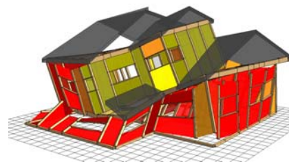
木造住宅の構造性能評価法のイメージ (地震応答シミュレーション)
