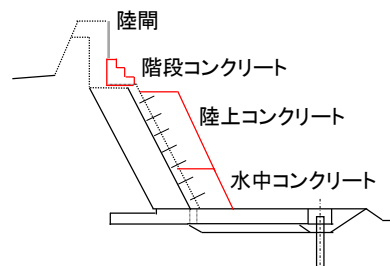
図-3.4(12) 階段コンクリートと陸間設置
