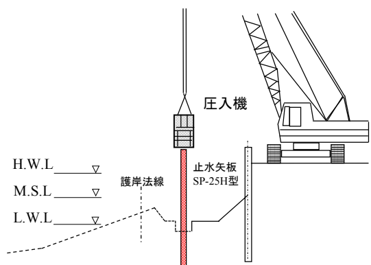
図-2.4(3) 基礎工 (止水矢板打設)
