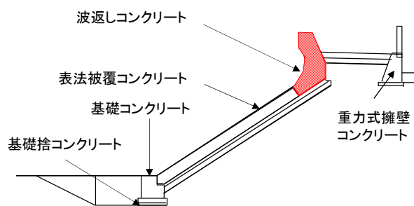
図 6.4(6) 波返しコンクリート
