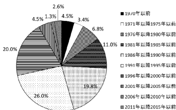
図-3.44 構造物築造系作業船の建造年割合
