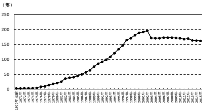
図-3.5 グラブ浚渫船隻数の推移
