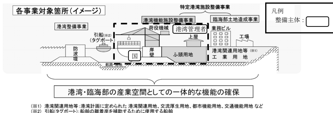
図-3 コンテナターミナルを構成する施設（岸壁、ふ頭用地、荷役機械等）の整備主体と事業方式 5) （公共方式で岸壁の整備主体が国の場合）
