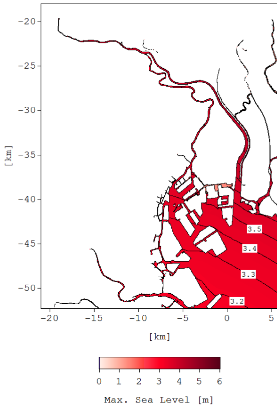
図-A.5 最高潮位 (海面上昇量: 0.40m)
