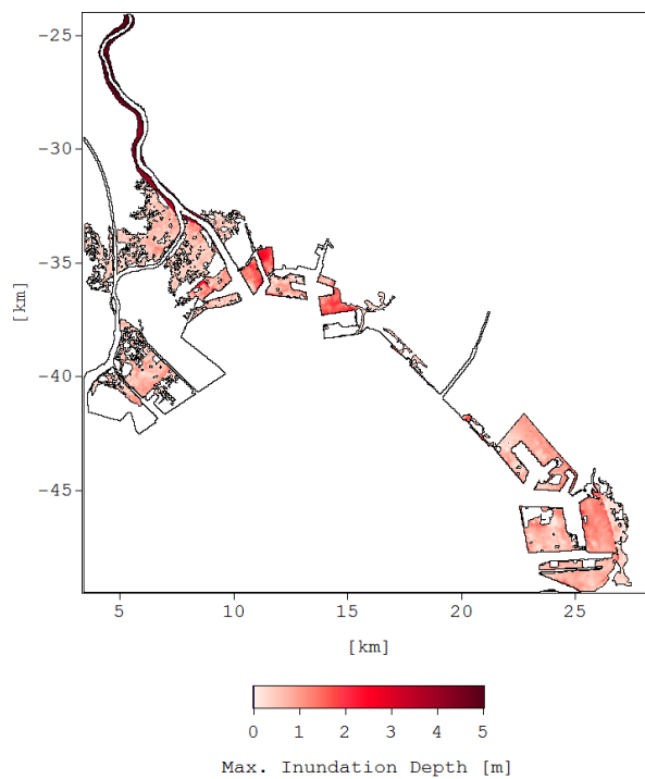
図-D.3 最大浸水深（海面上昇量：0.00m）
