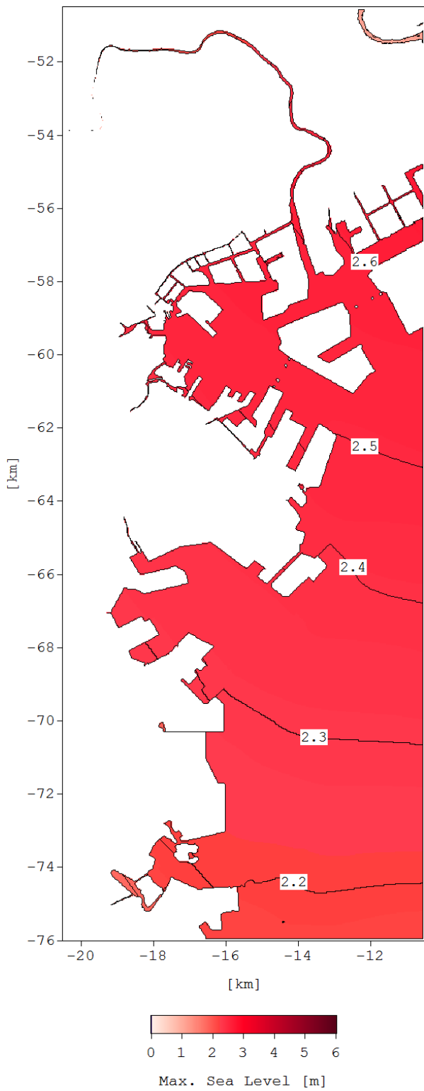
図-I.3 最高潮位 (海面上昇量: 0.20m)
