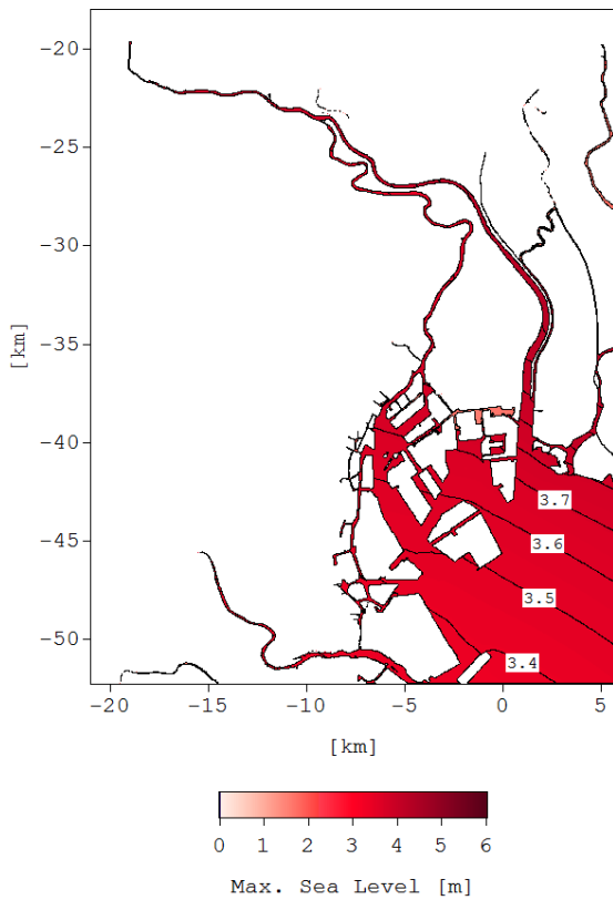
図-A.6 最高潮位 (海面上昇量: 0.60m)
