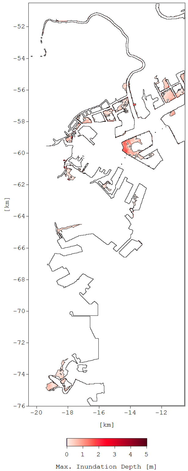
図-I.4 最大浸水深 (海面上昇量: 0.20m)
