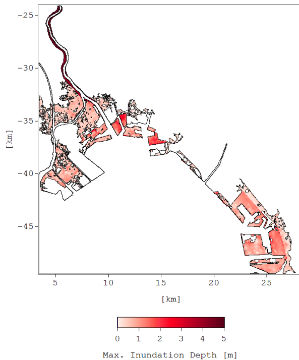
図-D.4 最大浸水深（海面上昇量：0.20m）
