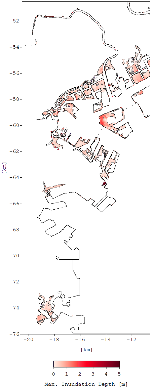
図-4.32 最大浸水深（横浜港地域） （海面水位上昇量 0.40m，河川流量なし）
