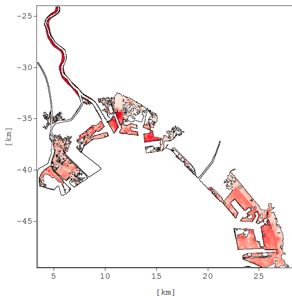
図-4.9 最大浸水深（千葉港地域北部） （海面水位上昇量 0.00m, 河川流量なし）
