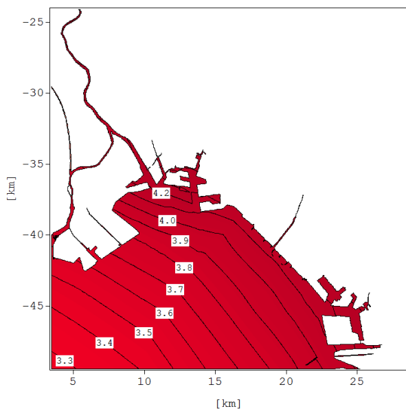
図-4.7 最高潮位（千葉港地域北部） （海面水位上昇量 0.00m, 河川流量なし）
