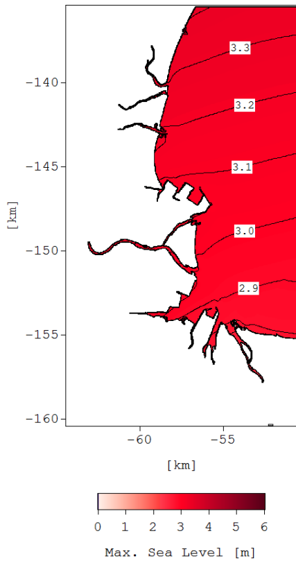
図-1.6 最高潮位（海面上昇量：0.60m）
