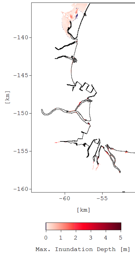
図-1.7 最大浸水深（海面上昇量：0.40m）
