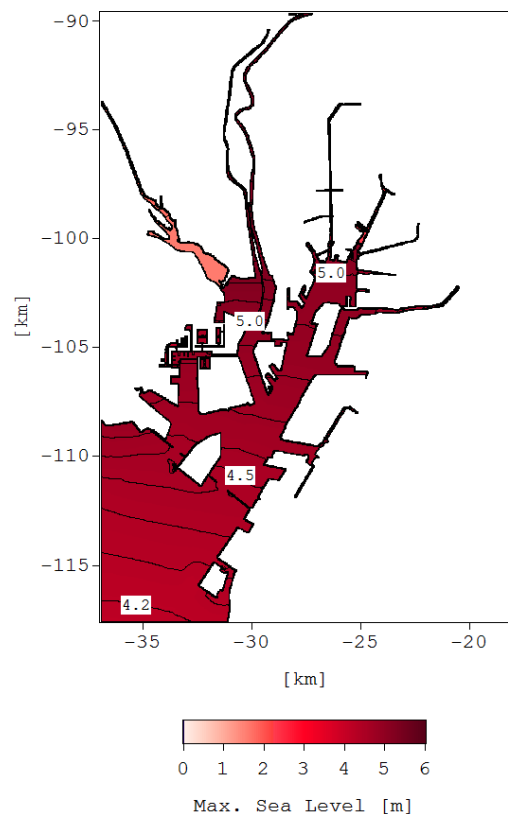
図-4.2 最高潮位（名古屋港地域） (海面水位上昇量 0.40m, 河川流量なし)
