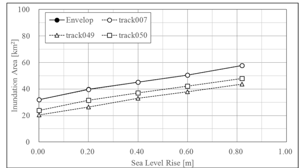
図-4.17 海面水位上昇量と浸水面積 （三河港地域）（河川流量なし）
