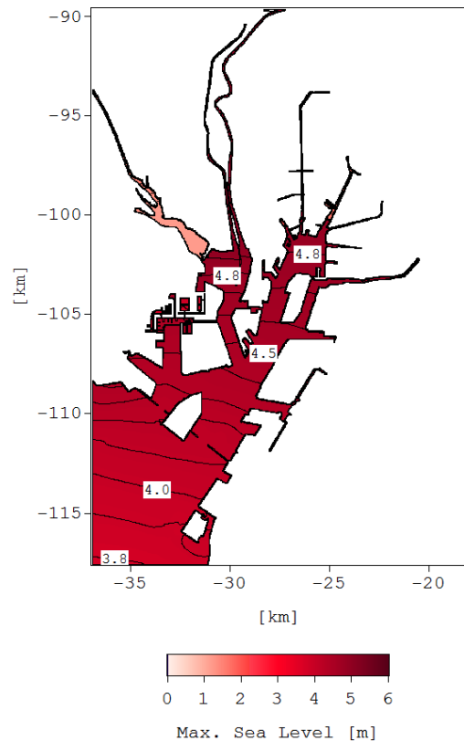
図-4.1 最高潮位（名古屋港地域） (海面水位上昇量 0.00m, 河川流量なし)
