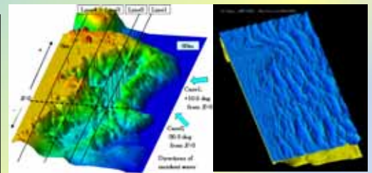
ブシネスクモデルによる波浪変形計算出力例
