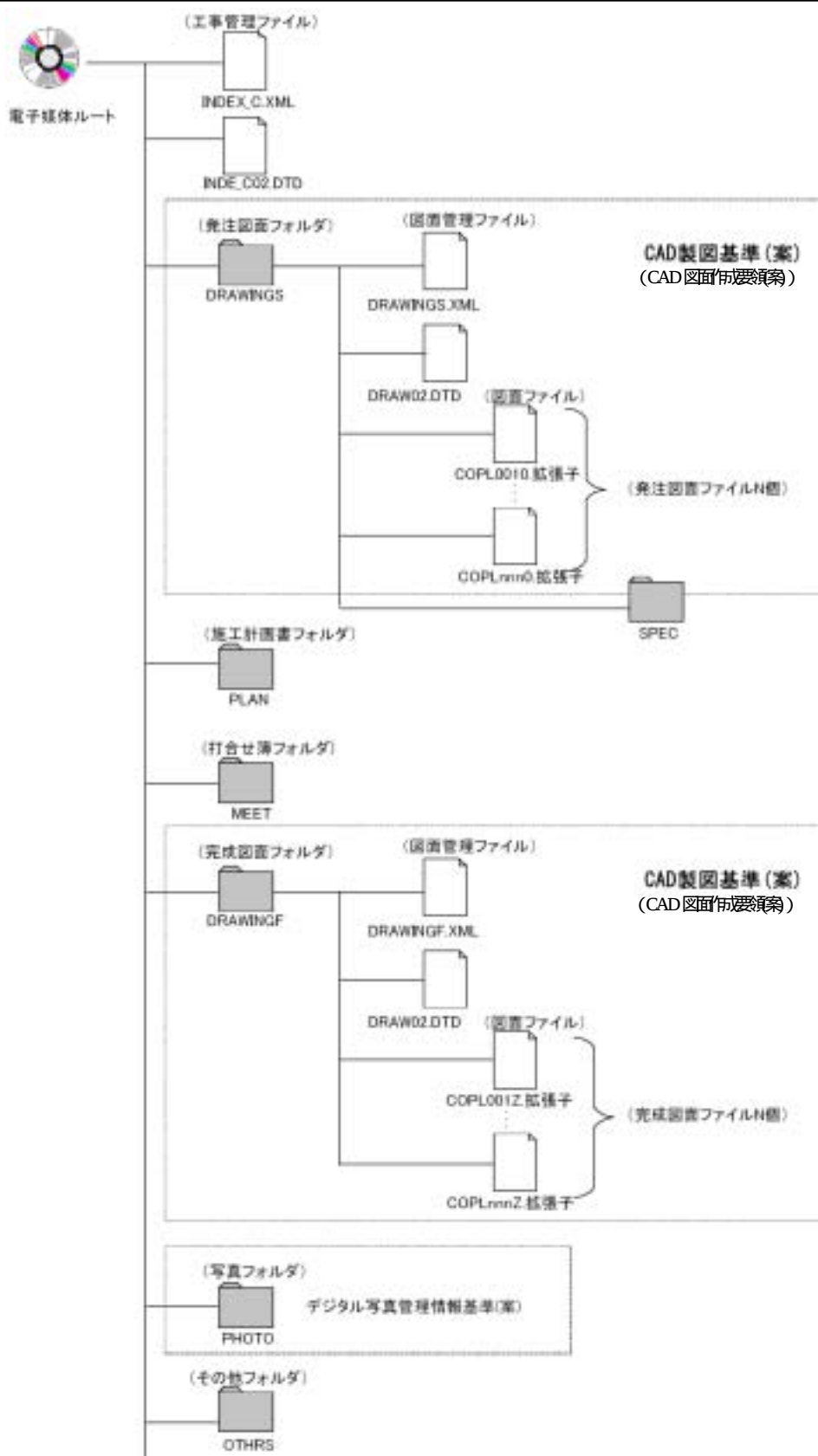
図 1-5 「工事完成図書の電子納品要領(案)」のフォルダ構成
