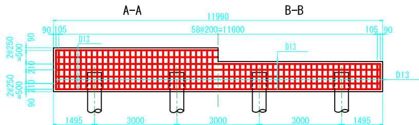
正面図
