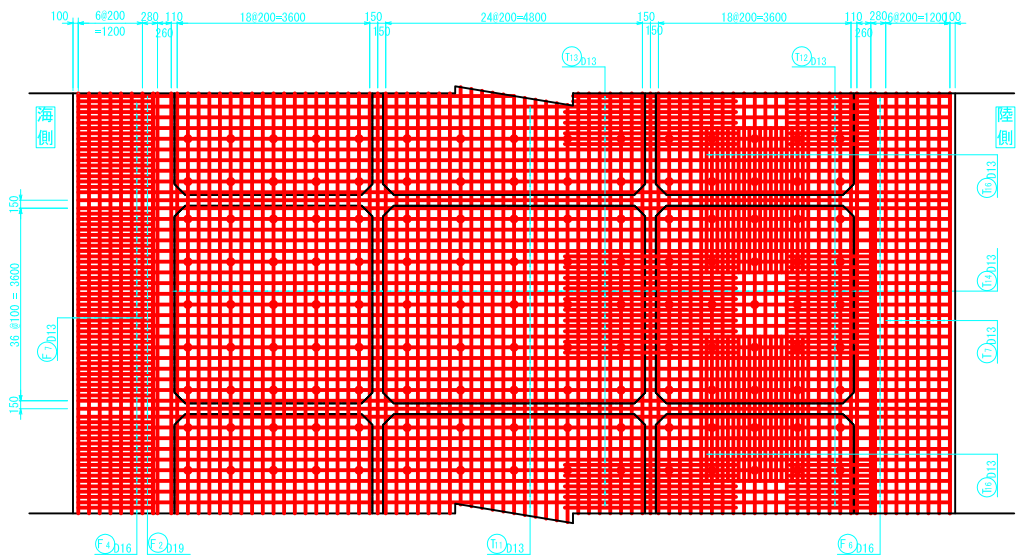
上 側
