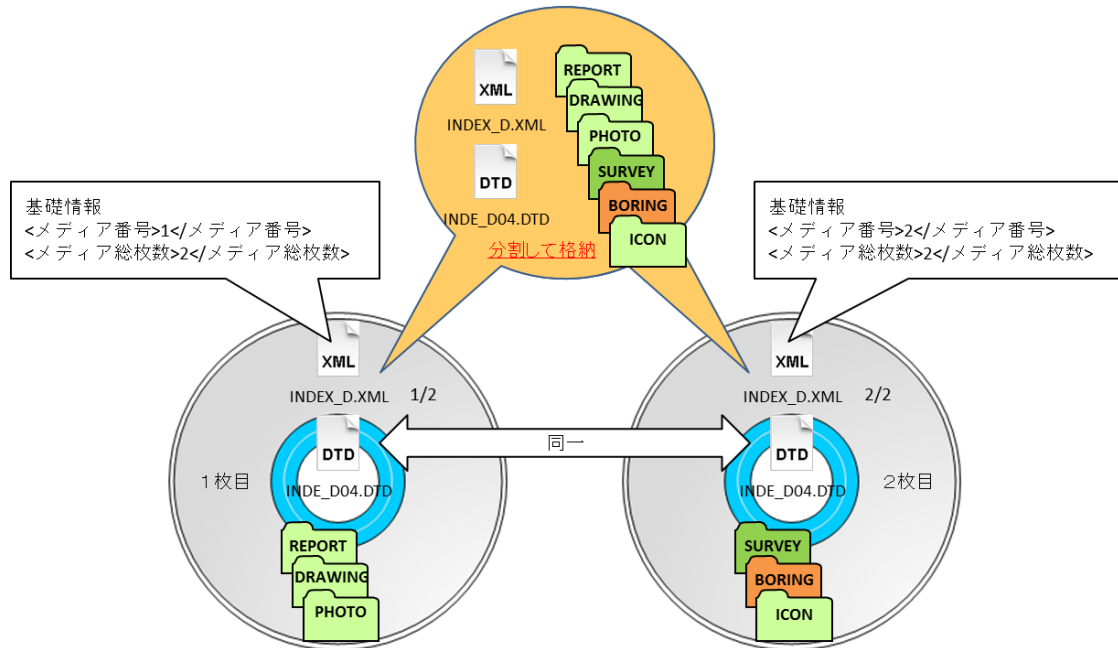
図 6-19 電子媒体が 2 枚になる場合の作成（例）
