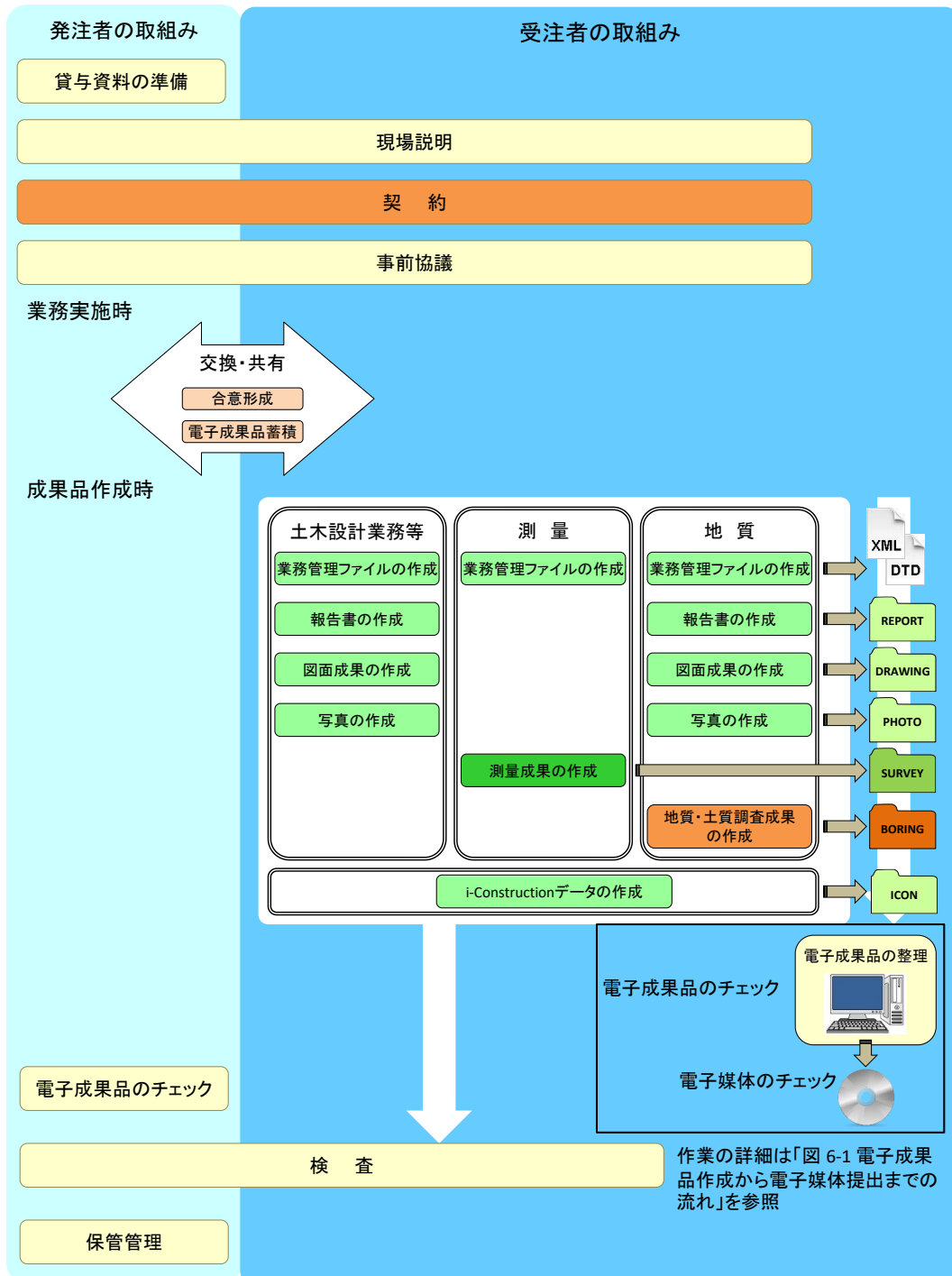
図 2-1 業務における電子納品の流れ
