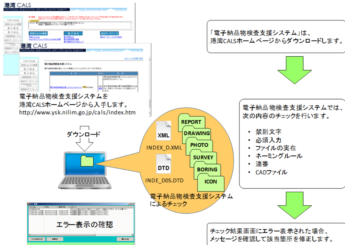
図 6-15 電子納品物検査支援システムを用いた電子成果品のチェック（例）
