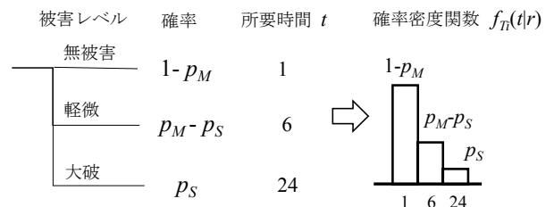
図-2 構成要素のイベントツリーと損傷確率、所要時間および確率密度関数
