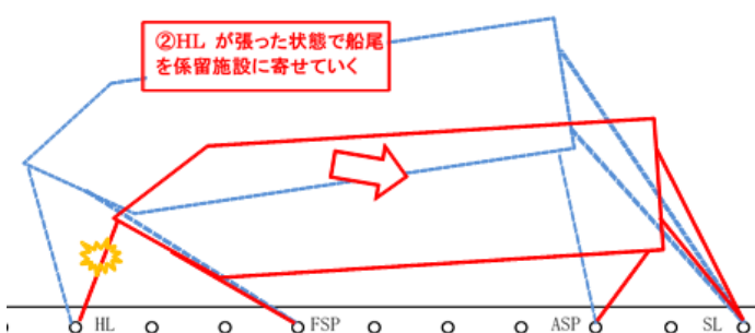
図 3.9 HL の破断事故のケース (②)
