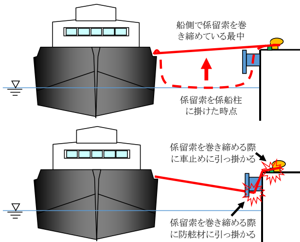
図 2.12 係留索の巻き締め状況
