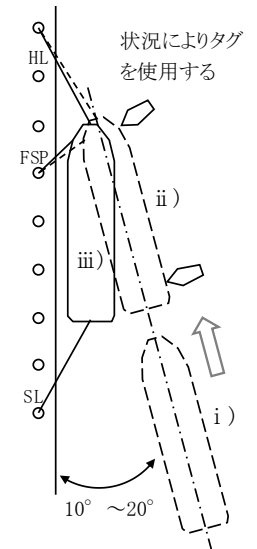
図 2.2 旧操船方法による入船接岸 ※文献6)を基に加筆
