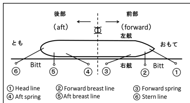
図2.1 係留索の取り方や名称 4)
