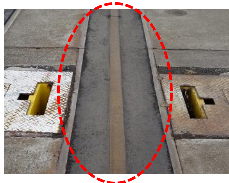
図 4.6 使用されなくなった荷役機械の溝を充填し平場を確保(安全性向上事例)
