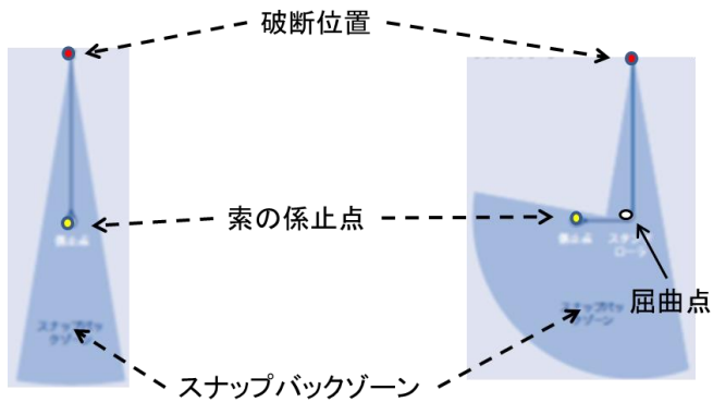
図 2.7 スナップバックゾーン ※文献 6)を基に加筆
