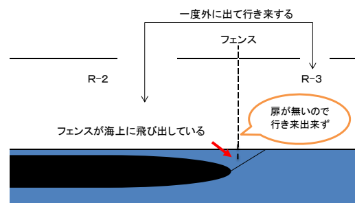
図 4.31 作業通路を確保できないフェンス
