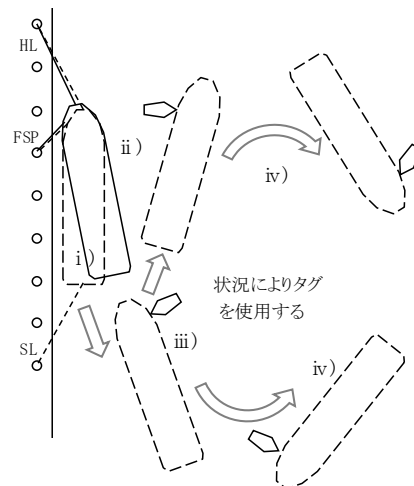
図 2.6 入船係留から係留索を利用したの離岸 ※文献 6) を基に加筆
