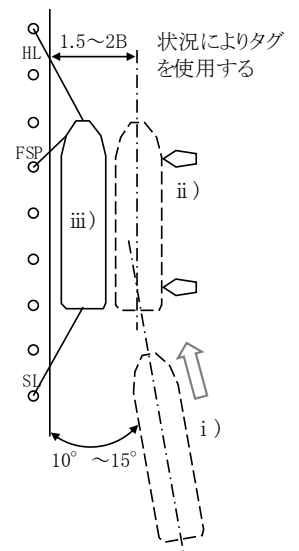
図 2.3 平行着岸による入船接岸 ※文献6)を基に加筆
