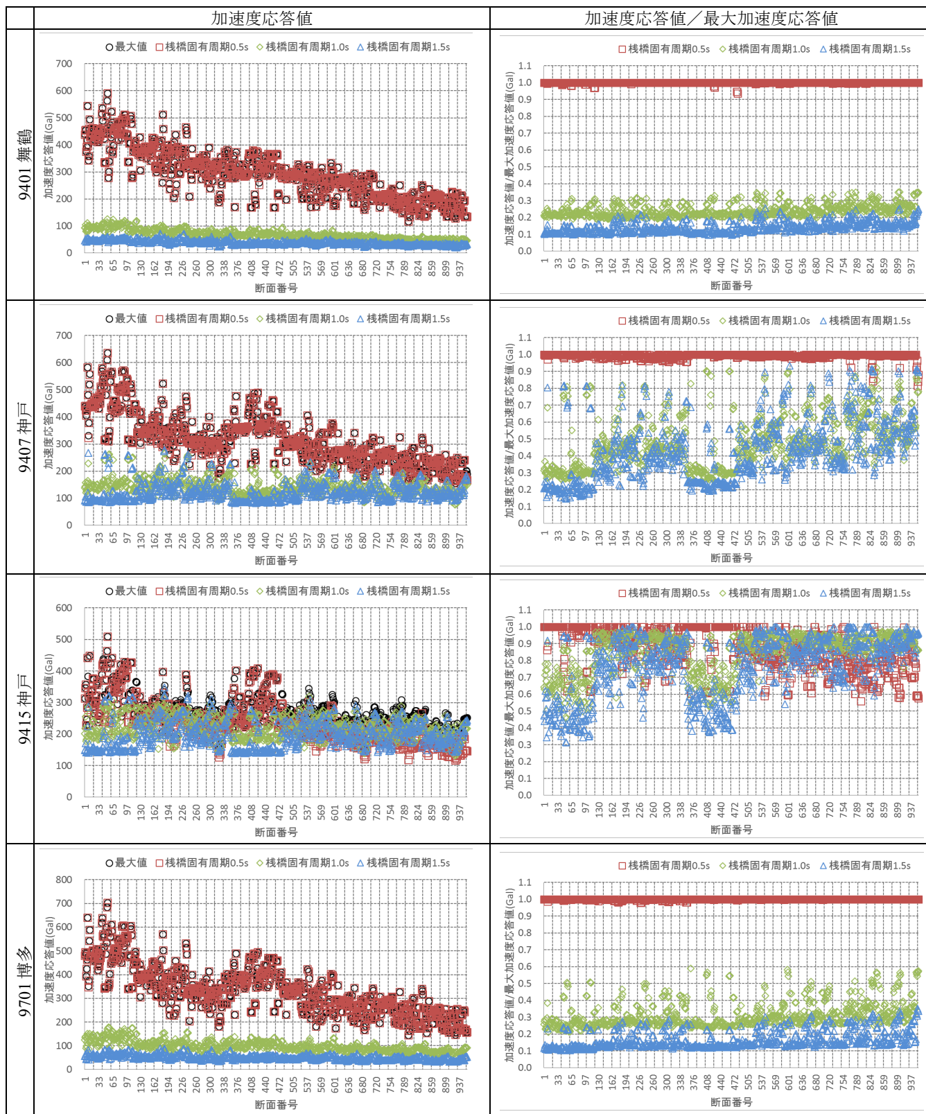
図-51 断面ごとの加速度応答値および加速度応答値と最大加速度応答値の比③
