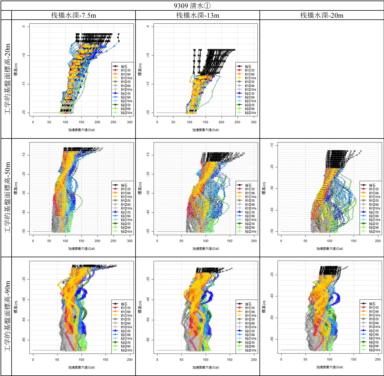
図-25 出力節点ごとの加速度最大値(入力地震動：9309 清水①)
