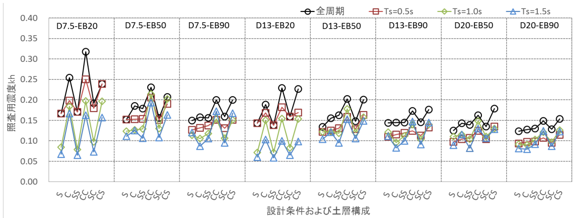
図-80 設計条件および土層構成ごとの照査用震度の最大値(9211 千葉)
