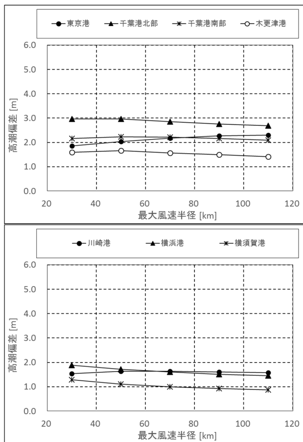
図-5.7 台風の最大風速半径と高潮偏差（東京湾）
