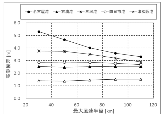
図-5.8 台風の最大風速半径と高潮偏差（伊勢湾）
