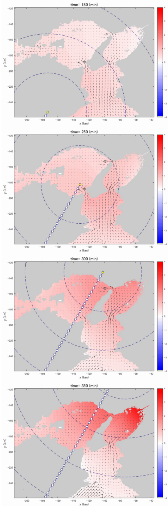
図-3.7 大阪湾の高潮伝播 (track009)
