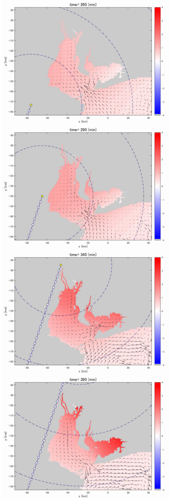
図-3.4 伊勢湾の高潮伝播 (track007)
