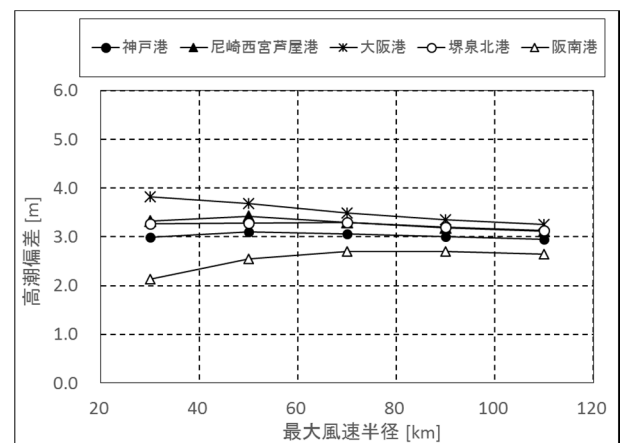
図-5.9 台風の最大風速半径と高潮偏差（大阪湾）
