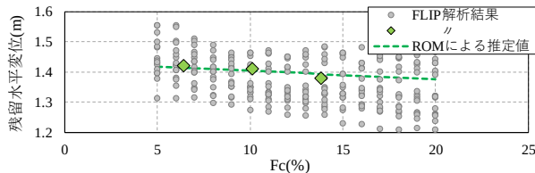
(b) 細粒分含有率Fcと残留水平変位量の関係
