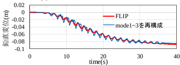
(b) 鉛直変位時刻歴 (岸壁先端)
