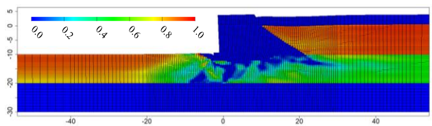
図-4.7 残留値スナップショット (CASE-5)
