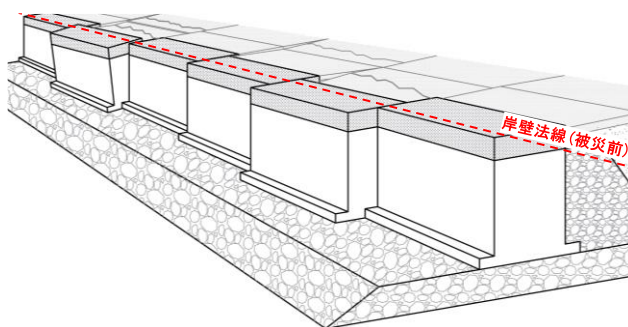
図-1.1 岸壁法線の出入りのイメージ
