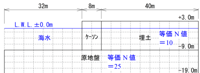
図-2.6 解析モデル(例題)
