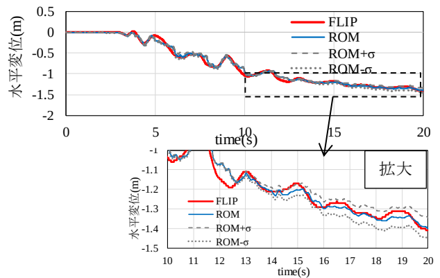
図-4.12 水平変位時刻歴（岸壁天端）
