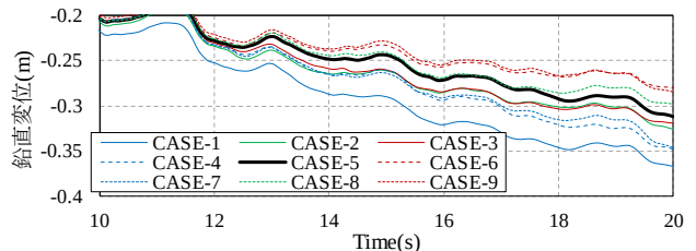
図-4.9 鉛直変位時刻歴
