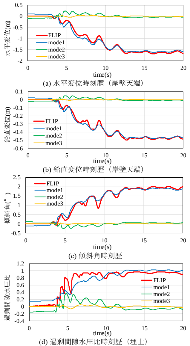
図-3.9 時刻歴応答値
