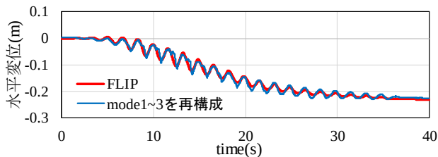
(a) 水平変位時刻歴 (岸壁先端)
