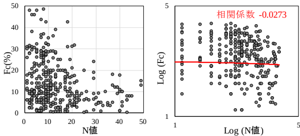
図-4.4 N値と細粒分含有率Fcの関係
