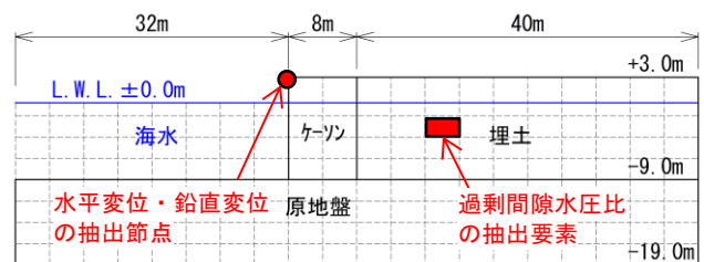
図-2.10 解析結果時刻歴抽出点
