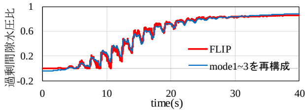
(c) 過剰間隙水圧比時刻歴 (埋土)
