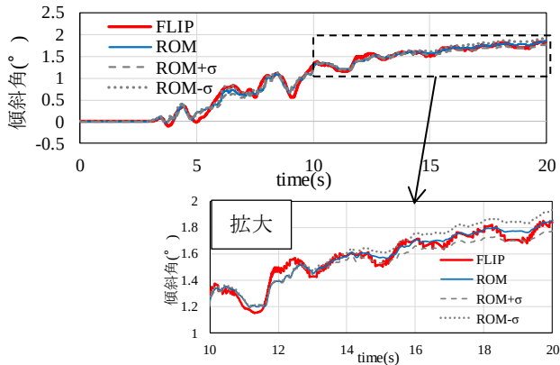
図-4.14 傾斜角時刻歴
