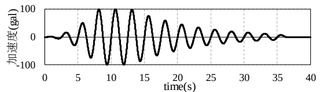
図-2.7 地震波形(例題)
