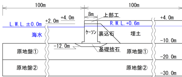
再掲図-3.1 解析モデル図
