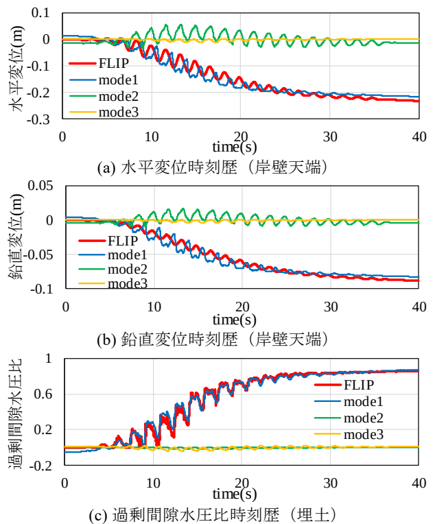
図-2.11 時刻歴応答値
