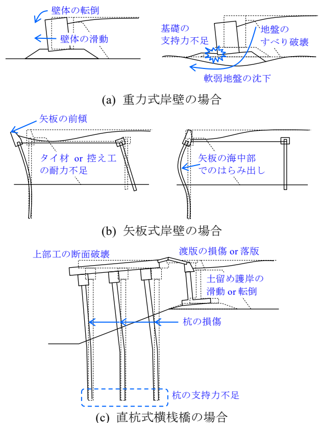
図-1.2 係留施設の破壊形態の例
