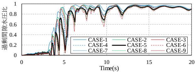
図-4.11 過剰間隙水圧比時刻歴
