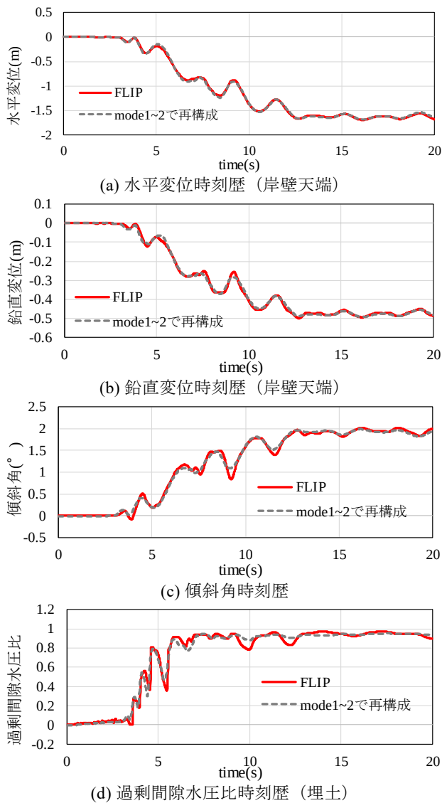
図-3.14 時刻歴応答値
