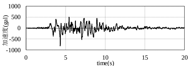
再掲図-3.4 神戸波
