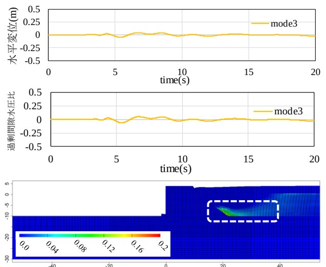
図-3.13 モード3が示す挙動
