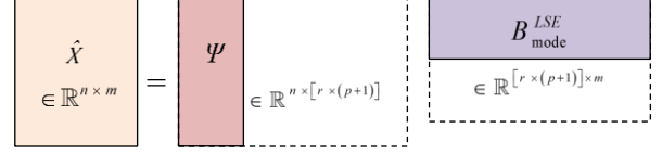
図-2.3 代替モデルの関係式概念図
