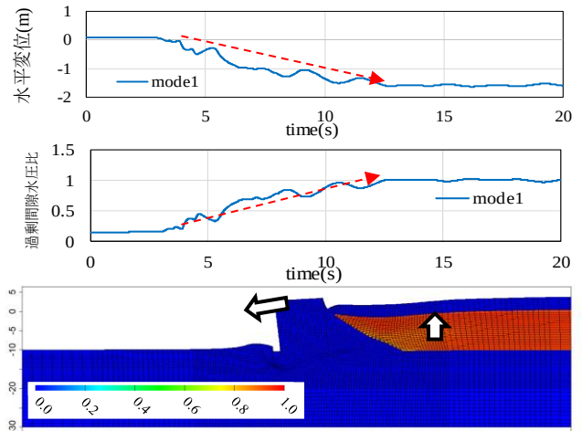
図-3.11 モード1が示す挙動
