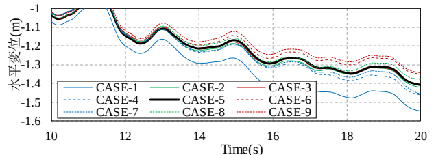
図-4.8 水平変位時刻歴
