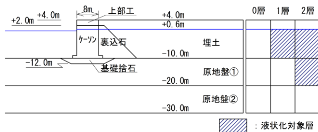
図-3.3 液状化対象層
