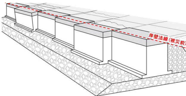
再掲図-1.1 岸壁法線の出入りのイメージ
