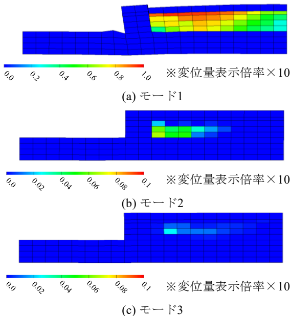
図-2.9 スナップショット（残留値）
