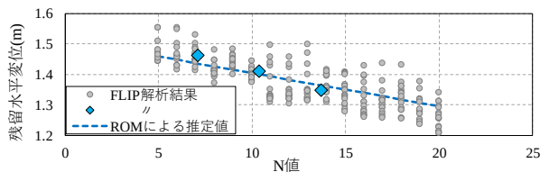
(a) N値と残留水平変位量の関係
