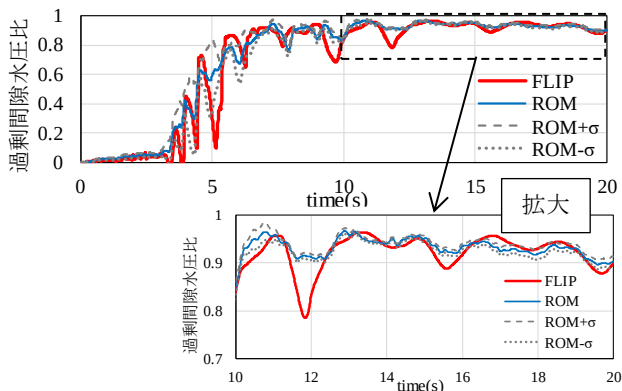
図-4.15 過剰間隙水圧比 (埋土)
