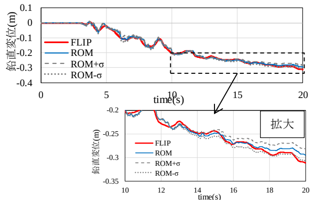
図-4.13 鉛直変位時刻歴（岸壁天端）
