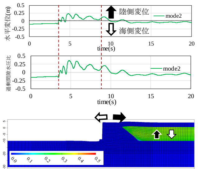
図-3.12 モード2が示す挙動
