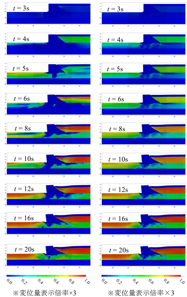
図-4.16 解析結果のスナップショット
