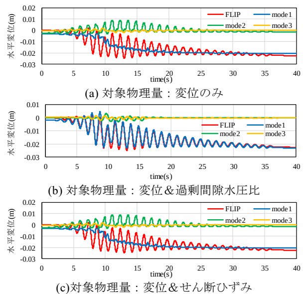
図-3.2 各モードにおける水平変位時刻歴
