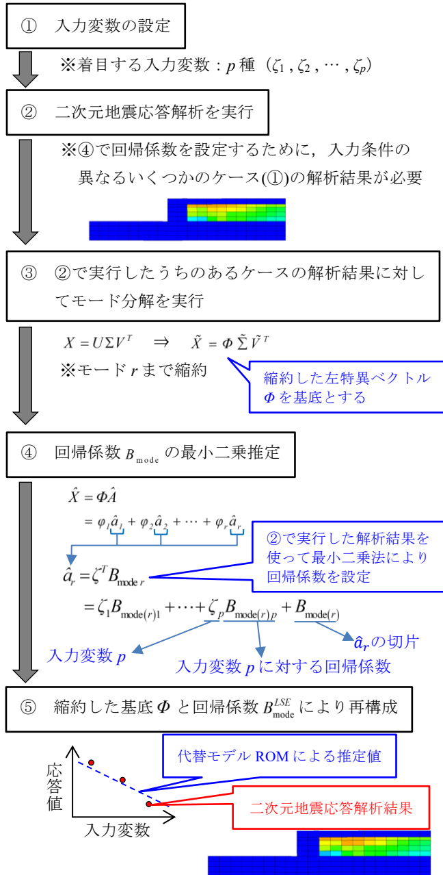
図-2.5 代替モデル構築のイメージ
