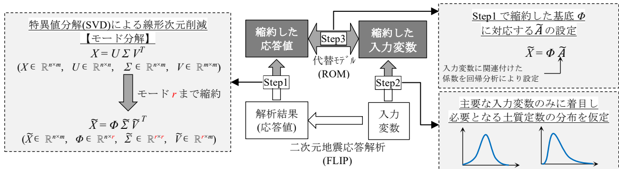
図-2.1 本研究で目指す代替モデル構築の全体構造
