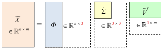
図-2.12 例題におけるモード分解のイメージ
