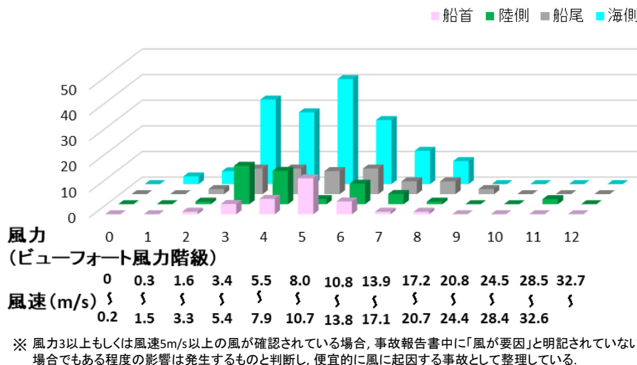
図-4.4 風に起因する事故発生時(離着岸時)の風向と風力
