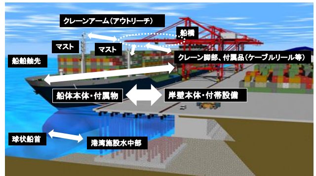
図-1.1 船舶の係留施設への衝突のイメージ
