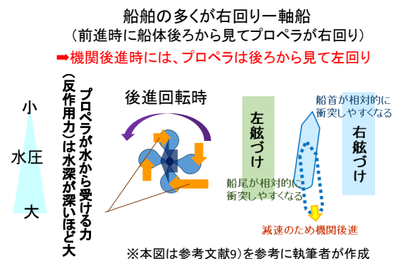
図-4.1 右回り一軸船の減速時挙動特性
