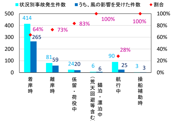
図-3.2 船舶の事故状況と風の影響
