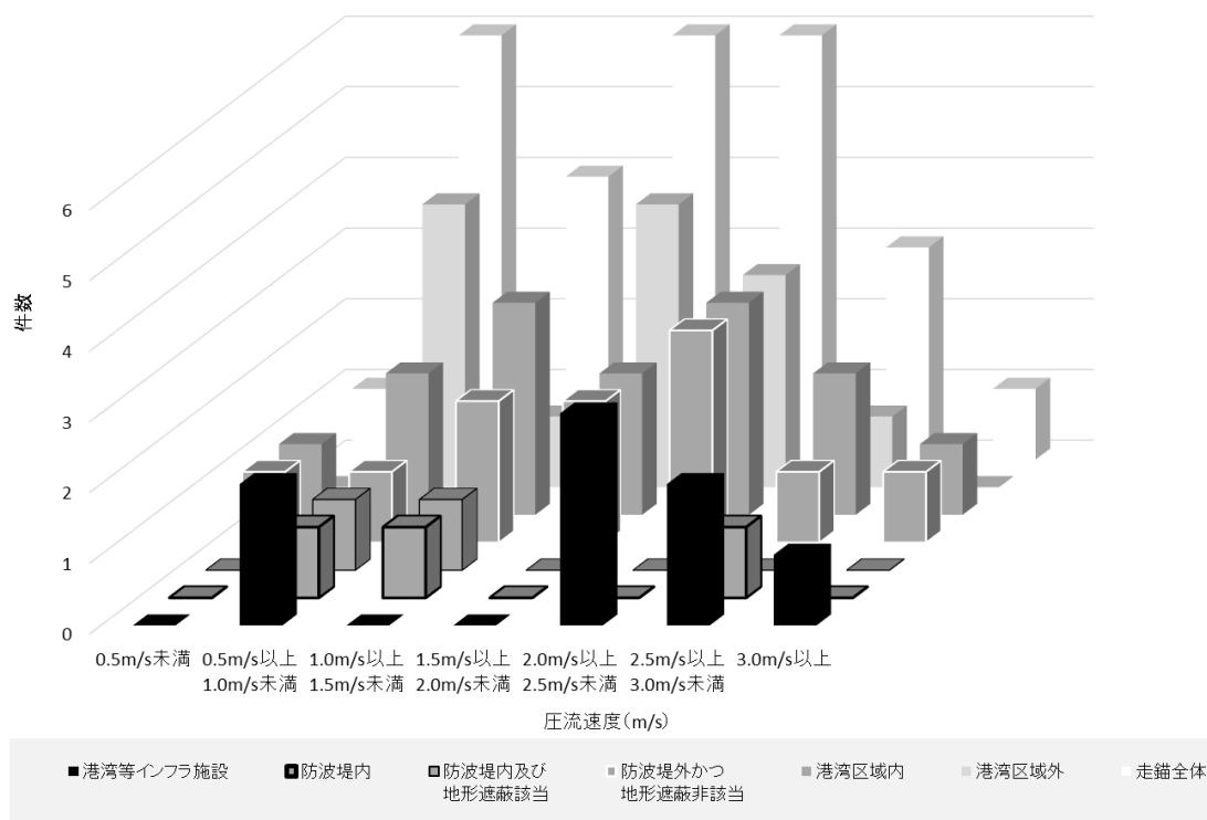
圧流速度分布図 (錨鎖使用のみ)
