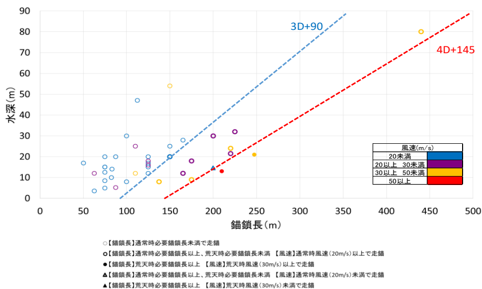
図-4.5 対象データの錨鎖式への適用
