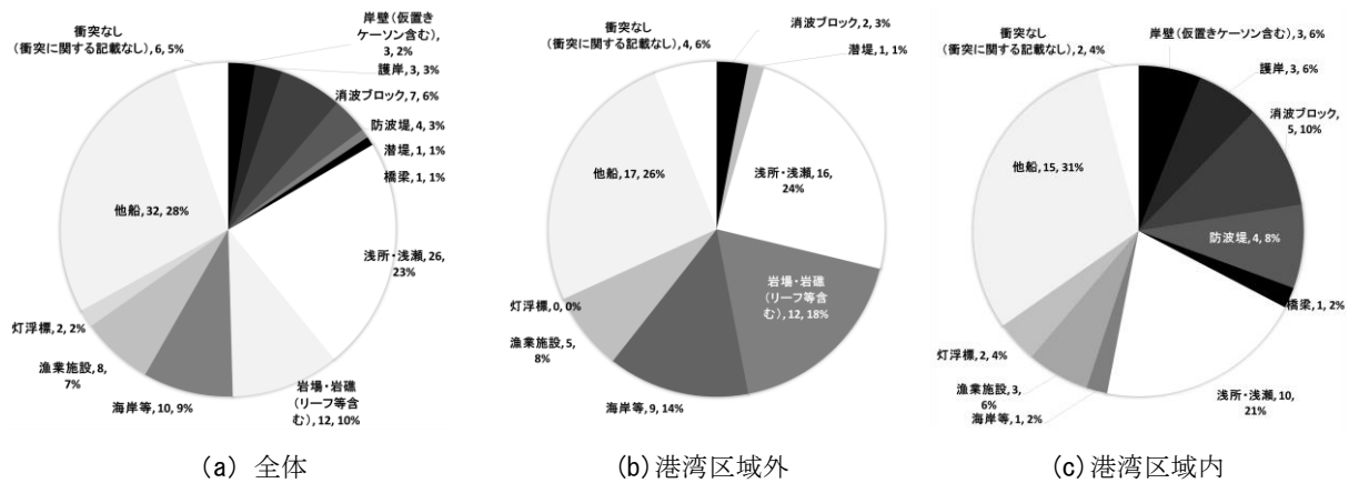
図-4.4 走錨・圧流後の乗揚・衝突施設
