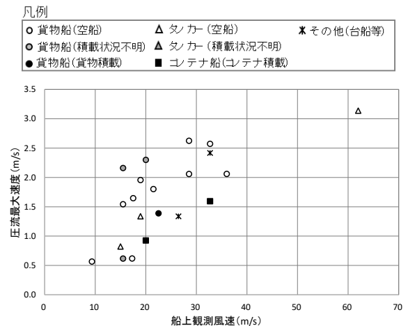
(a) 船上観測風速と圧流速度の関係
