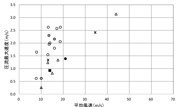
(c) 平均風速と圧流速度の関係
