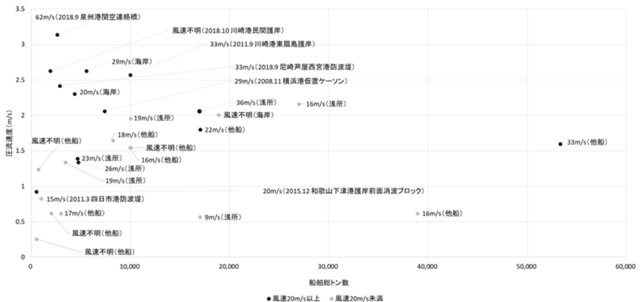
図-4.7 各風速の相関
