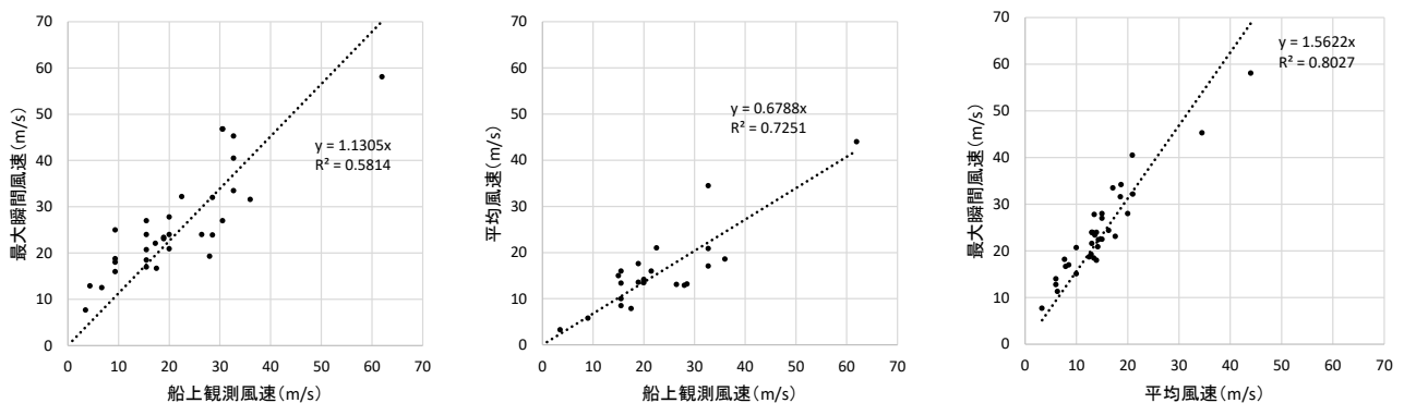
(a) 船上観測風速と最大瞬間風速の相関 (b) 船上観測風速と平均風速の相関 (c) 平均風速と最大瞬間風速の相関
