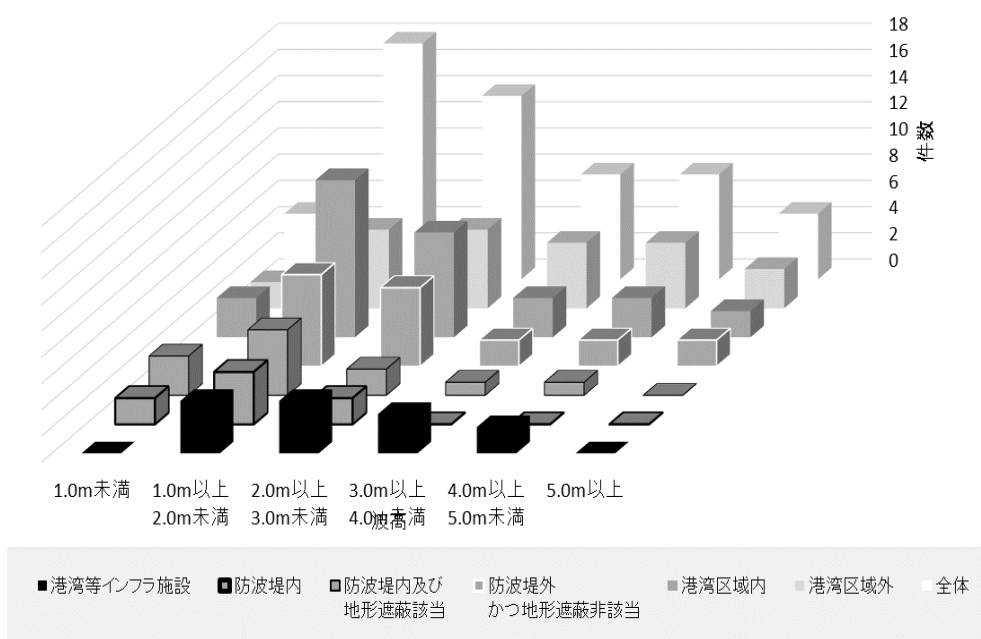
波高分布図 (錨鎖使用のみ)
