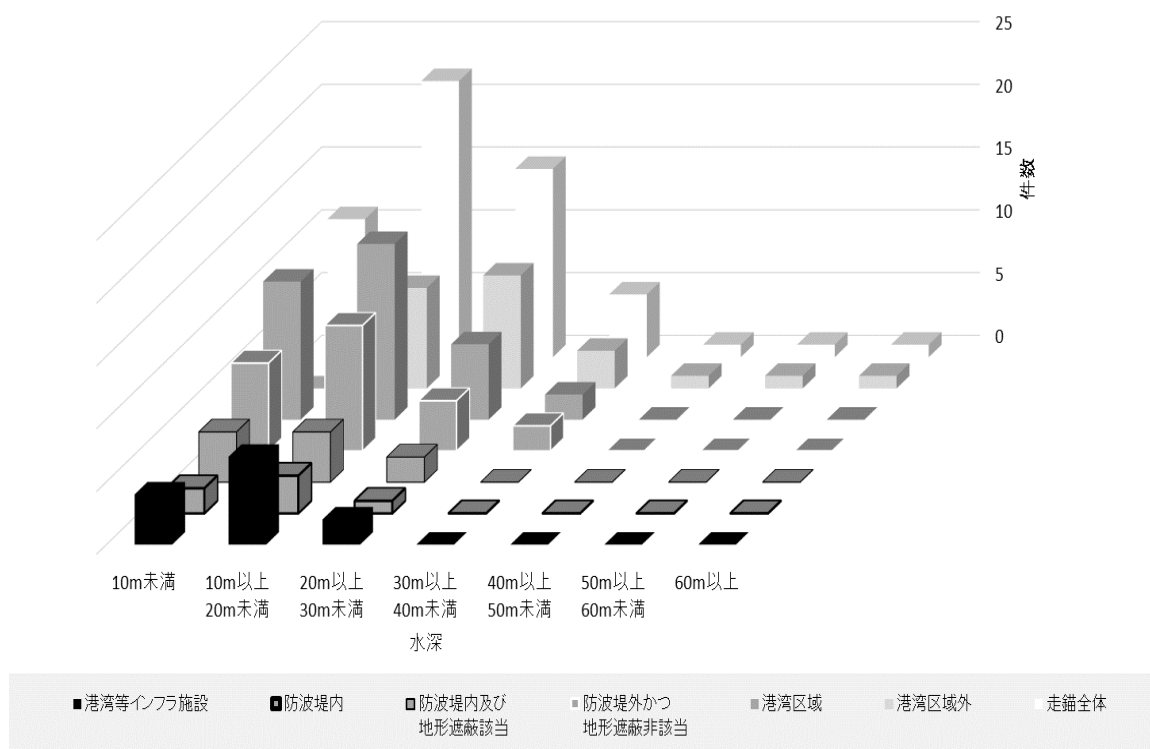
水深分布図 (錨鎖使用のみ)
