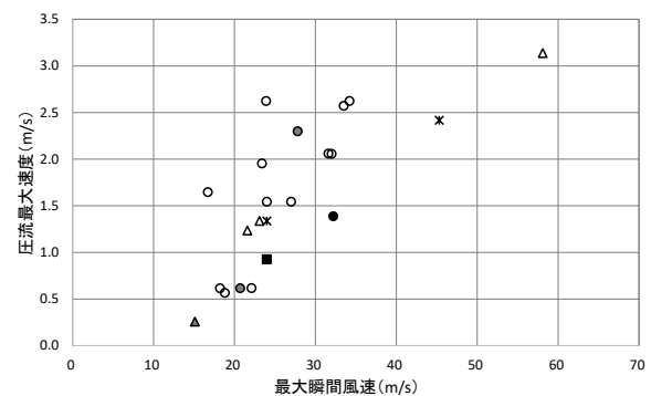
(b) 最大瞬間風速と圧流速度の関係
