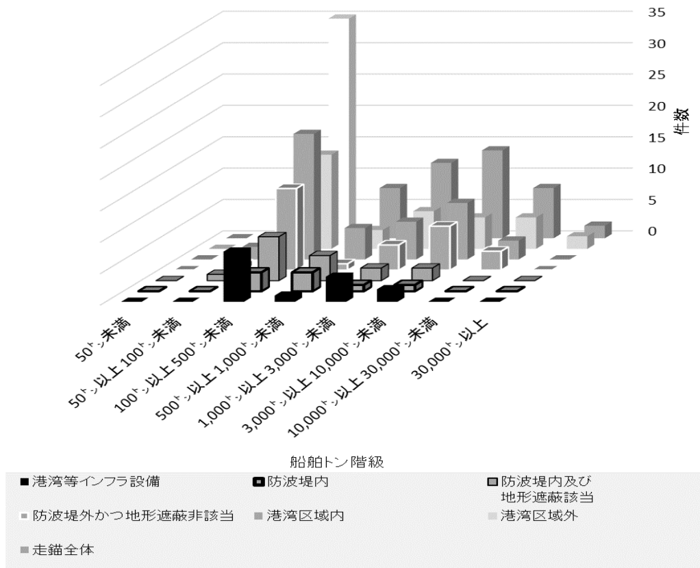
船舶トン数分布図 (錨鎖使用のみ)
