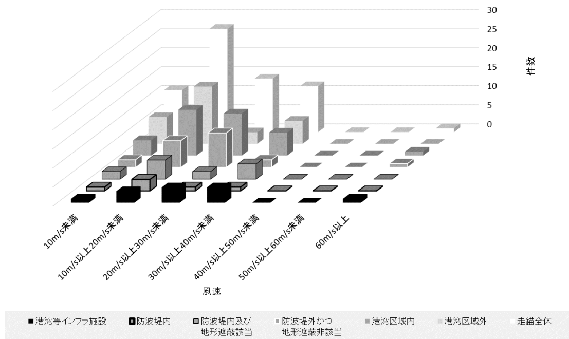
船上観測風速分布図 (錨鎖使用のみ)
