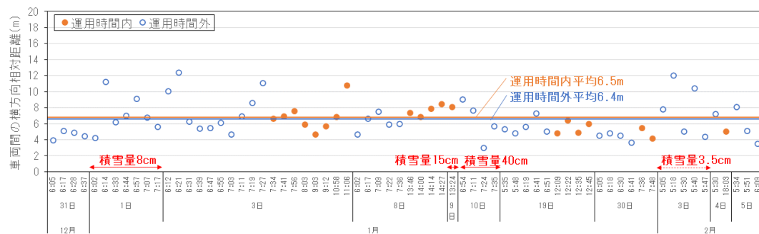
図-22 雁行隊列横方向の相対距離（スイーパー）
