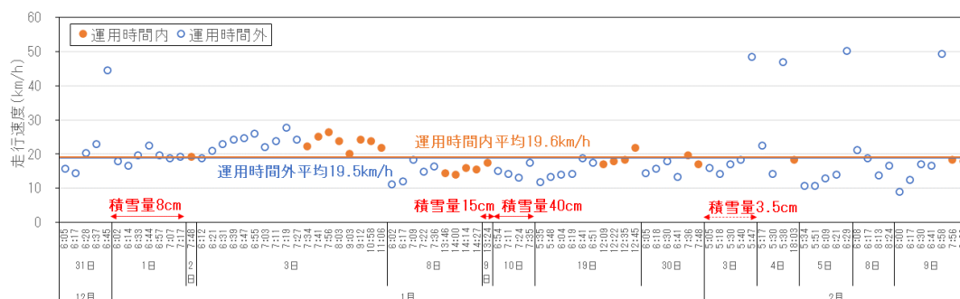
図-26 滑走路中間部での雁行隊列先頭車両の平均走行速度 (スイーパー)
