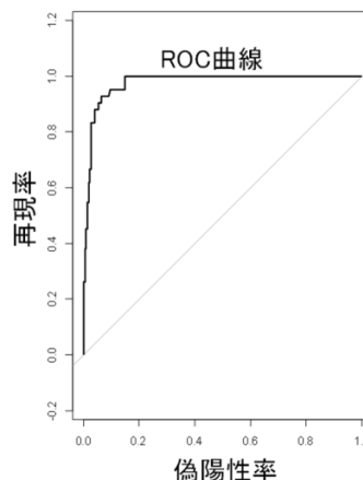
図-10 対象 FC の ROC 曲線
