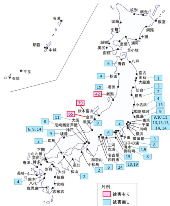
図-1 港湾地域強震観測網と令和6年能登半島地震で得られた地表面における速度PSI値( \text{cm/s}^{0.5} )
