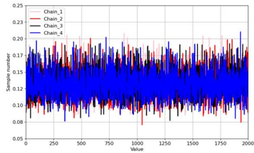
(b)パラメータ \beta_1 の結果
