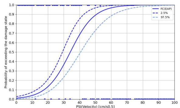
図-9 地震 fragility 曲線(係留施設を対象とした速度 PSI 値を指標とした港湾単位での被害発生確率)
