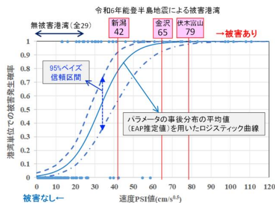
(b) 地震フラジリティ曲線
