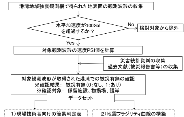
図-2 データ整理方法の概要
