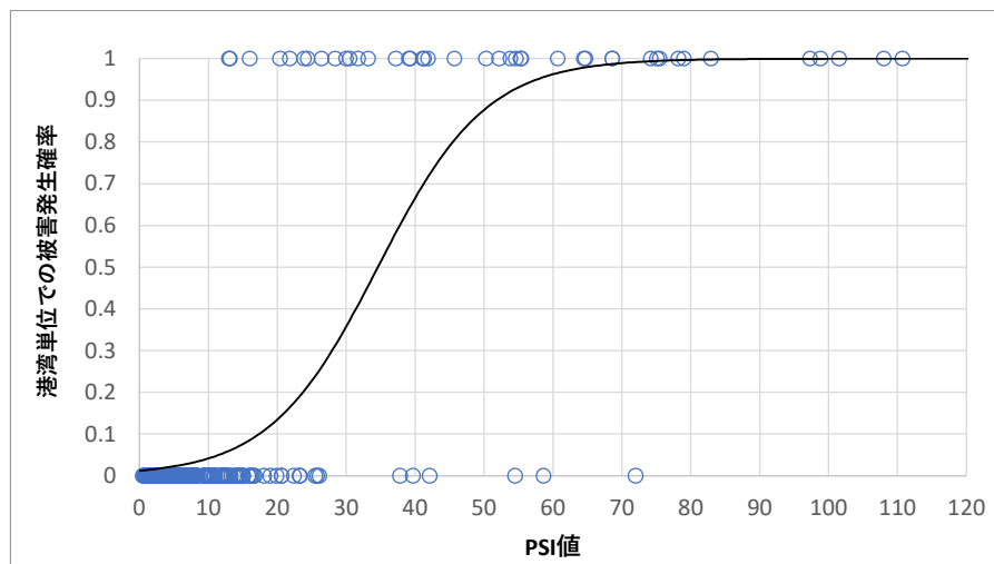
図-E.3 最尤法による地震 fragility 曲線 (係留施設を対象とした港湾単位での速度 PSI 値を指標とした被害発生確率)
