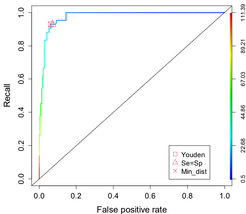
図-F.1 ROC曲線. ROC曲線の色は対応するカットオフ値（速度PSI値）を表す. 赤色のシンボルは3種類の方法（Youden's index method, Sensitivity equal to specificity methodおよびROC01 method）で決定されたカットオフ値の位置を表す.
