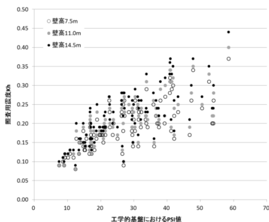
図-6 工学的基盤における速度 PSI 値と重力式岸壁の照査用震度との関係(背後地盤の固有周期 0.8s) 39)
