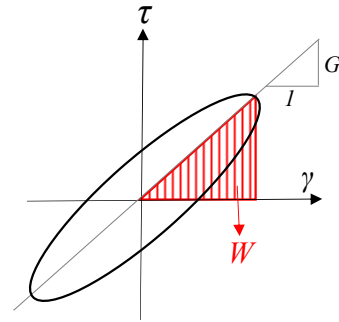
図-A.2 土要素のせん断応力とせん断ひずみの関係
