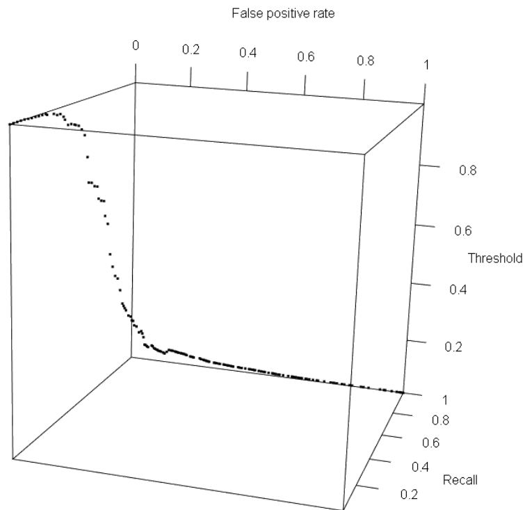
図-F.2 再現率 (Recall) , 偽陽性率 (False positive rate) , 閾値 (Threshold) の関係を表す3次元プロット図. キューブ上面から見ると, ROC曲線が確認できる.
