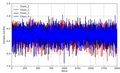
(a)パラメータ \beta_0 の結果
