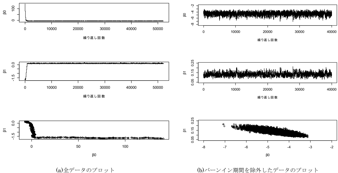
図-E. 6 RWHM 法による計算結果
