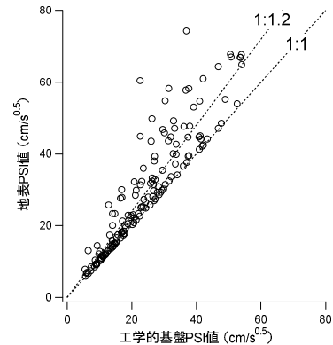
図-7 工学的基盤と地表での速度PSI値の関係 40)
