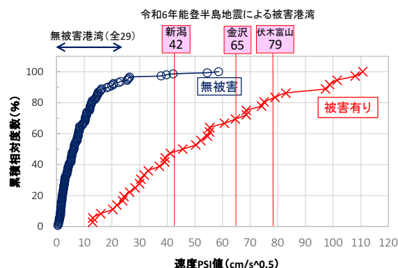
(a)「無被害港湾」と「被害港湾」の累積相対度数分布
