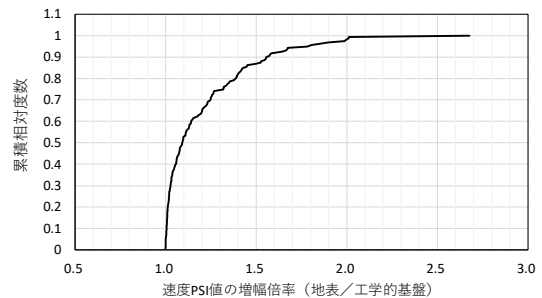
図-8 速度PSI値の増幅倍率（地表面／工学的基盤）の累積相対度数分布 40) より作成
