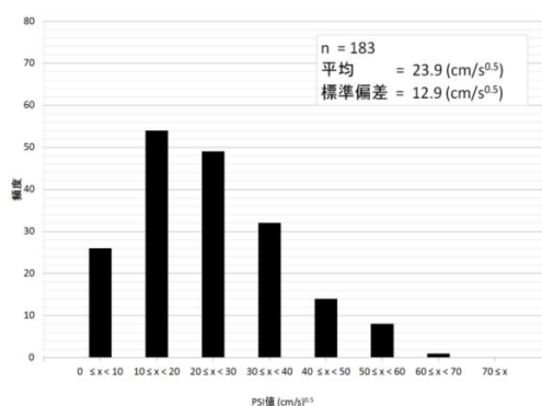
図-5 全国港湾のレベル1地震動（工学的基盤 2E 波）の速度 PSI 値の度数分布 39)
