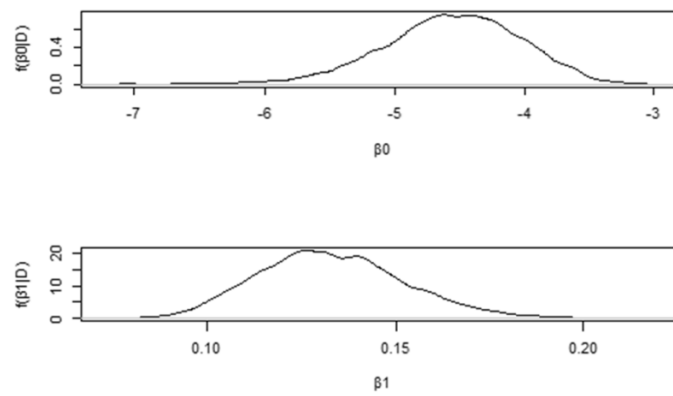
図-E.7 パラメータの事後分布
